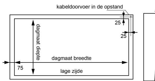
Maatvoering kabeldoorvoer in de opstand bij 75 mm opstanddikte
